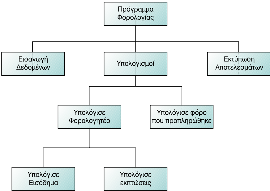
Σχ. 6.4. Ένα απλό δένδρο δομημένου προγράμματος
