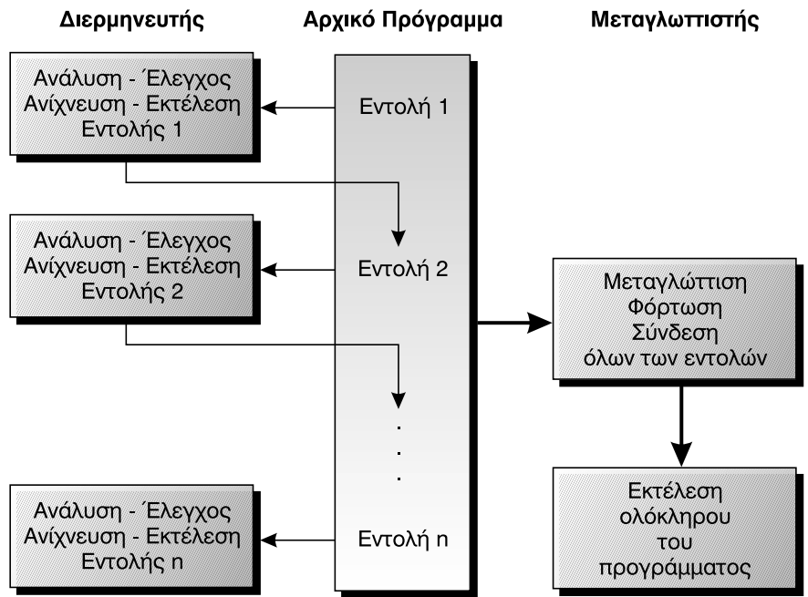
Σχ. 6.6. Διάγραμμα που συγκρίνει τον τρόπο εκτέλεσης ενός προγράμματος με τη χρήση διερμηνευτή και μεταγλωττιστή.
